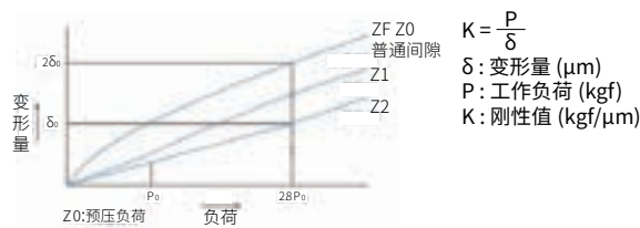
图 1.10.2 刚性数据
