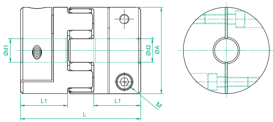
SRJ 可挠性联轴器规格表
