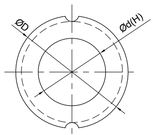
空心花键轴
