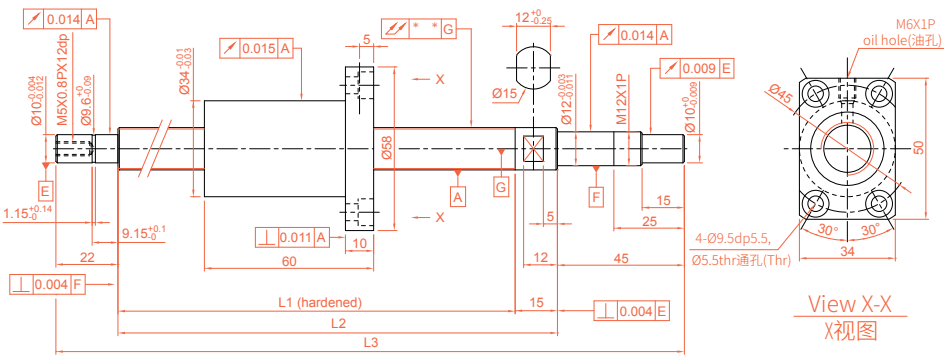
XSVR01520-01 精密研磨级系列规格尺寸表（研磨级轴端完成品）
