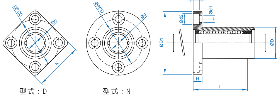
LF-L 系列规格尺寸表 ( 法兰式加长型 )
