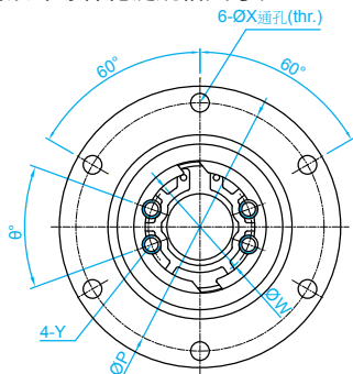
RBLY 精密滚珠螺杆花键规格尺寸表
