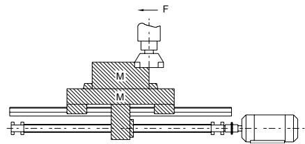
图 1.5.1 负荷惯性矩
