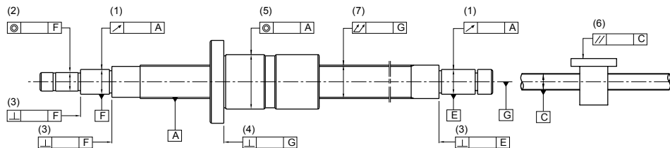
图 1.3.2 滚珠螺杆安装部位的精度 (ISO 3408)
