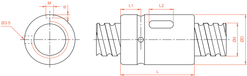
SCNI/SCI 精密研磨级系列规格尺寸表
