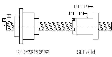
图 1.2.2 RBLY 系列
