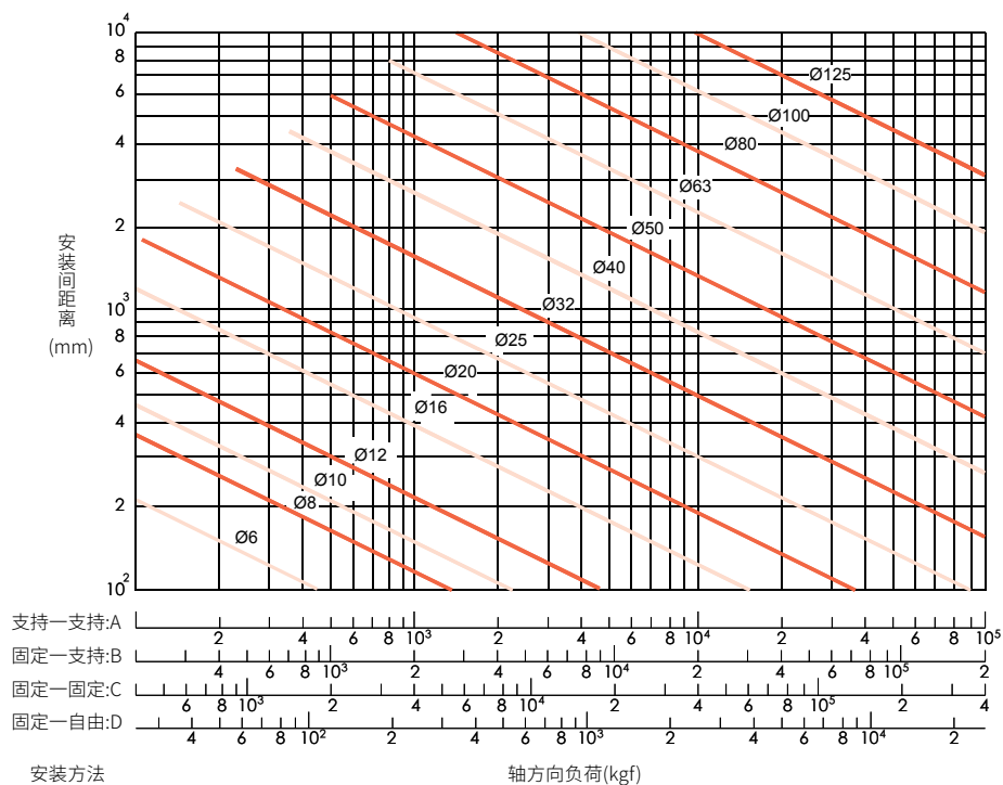
图 1.4.16 屈扭之容许压缩负荷
