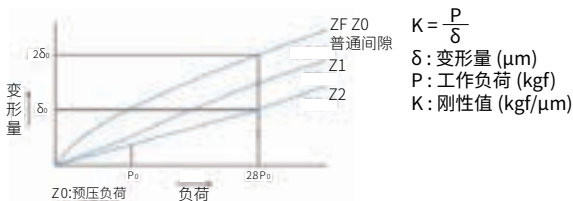
图 1.10.2 刚性数据
