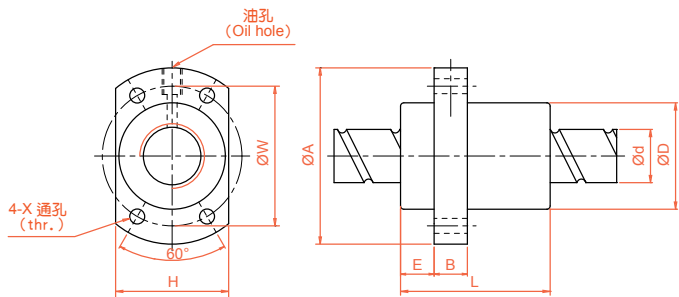
SFYA 转造级系列规格尺寸表
